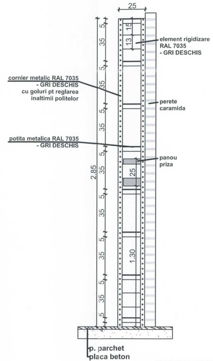
VEDERE LATERALA scara 1:20
