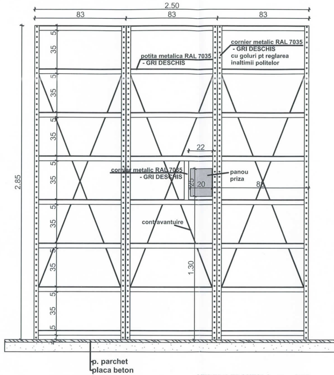
VEDERE FRONTALA scara 1:20
