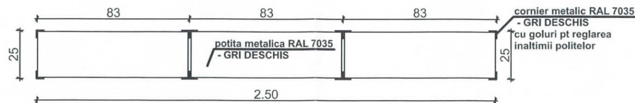
VEDERE ORIZONTALA scara 1:20
